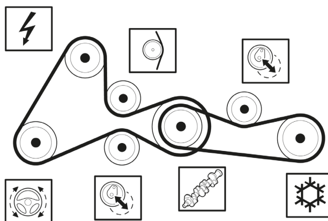
Fig. 1: Transmissão do grupo auxiliar em motores com número 0113089 ou inferior com polia tensora
