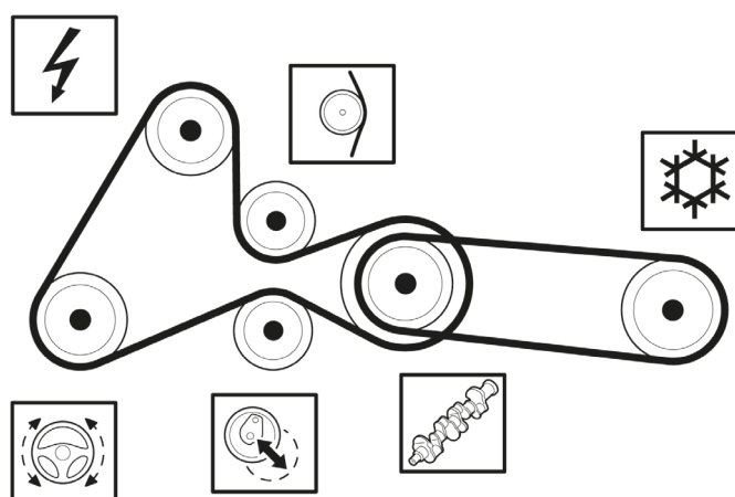
Fig. 2: Transmissão do grupo auxiliar em motores com número 0113090 ou superior com correia trapezoidal elástica
