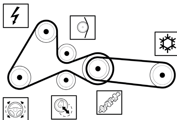
Figura 2: Transmisia auxiliară începând de la motorul nr. 0113090 cu curea elastică cu nervuri în V
