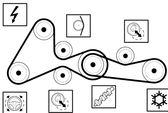
Figura 1: Transmisia auxiliară până la motorul nr. 0113089 cu folie întinzător
