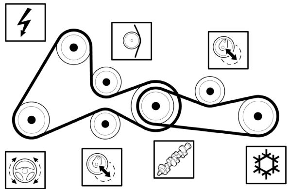
Зображення 1: Привод допоміжних агрегатів до номера двигуна 0113089 з натяжним роликом
