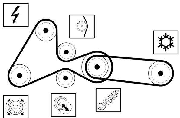
Зображення 2: Привод допоміжних агрегатів до номера двигуна 0113090 з еластичним поліклиновим ремнем
