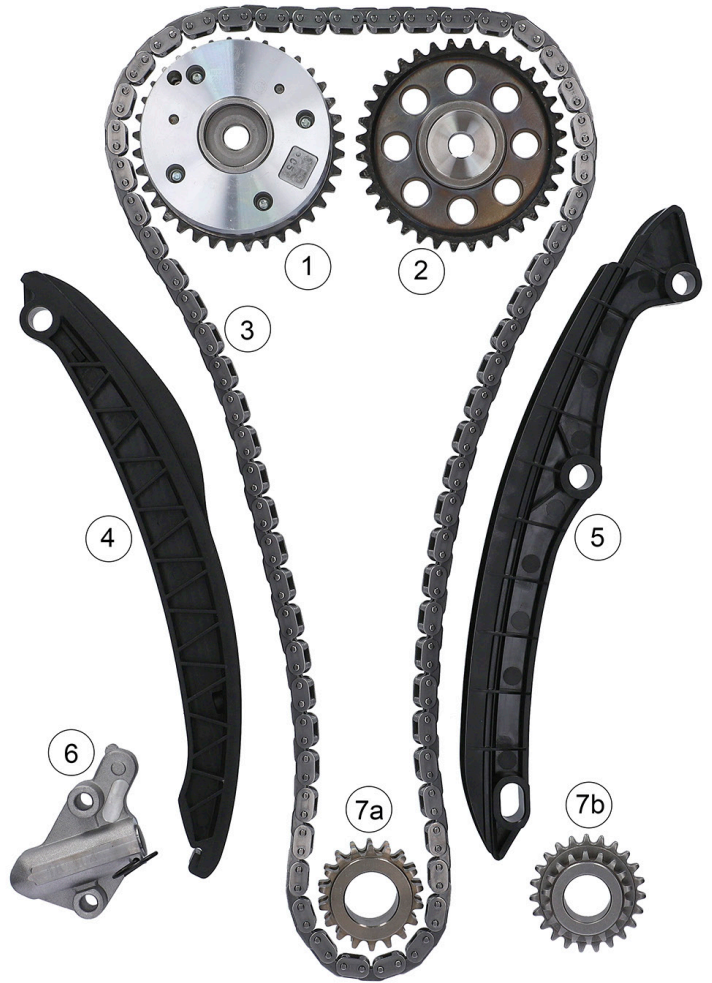
Kuva 1: 559 0154 30/559 0154 31 – jakoketjusarjan rakenneosat
