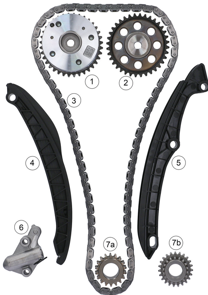
Figura 1: 559 0154 30/559 0154 31 – Componenti KIT catena di distribuzione
