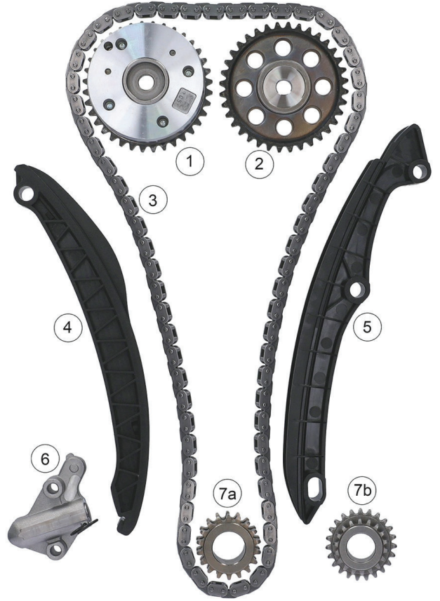
Resim 1: 559 0154 30/559 0154 31 – Zamanlama zinciri kiti bileşenleri
