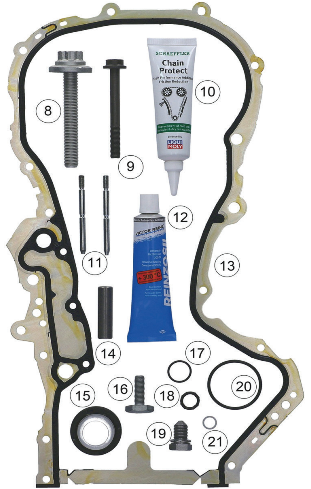
Resim 2: 559 0154 30/559 0154 31 - Zamanlama zinciri kiti ek parçaları
