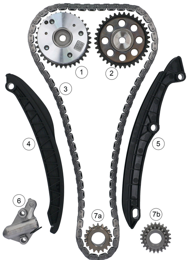
Зображення 1: 559 0154 30/559 0154 31 – Компоненти комплекту ланцюгового привода ГРМ
