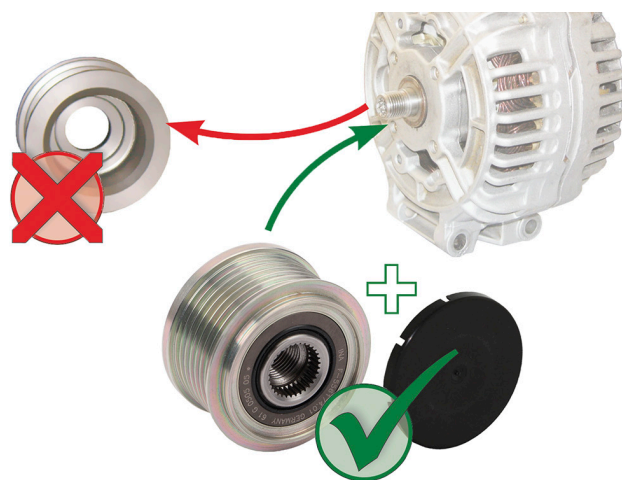
Výměna pevné řemenice za alternátorovou volnoběžku
