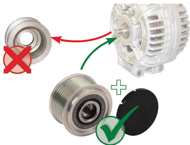
Trecerea de la fulia rigidă la o rolă unisens a alternatorului
