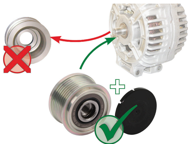
Заміна жорсткого шківів на шків генератора з обгінною муфтою
