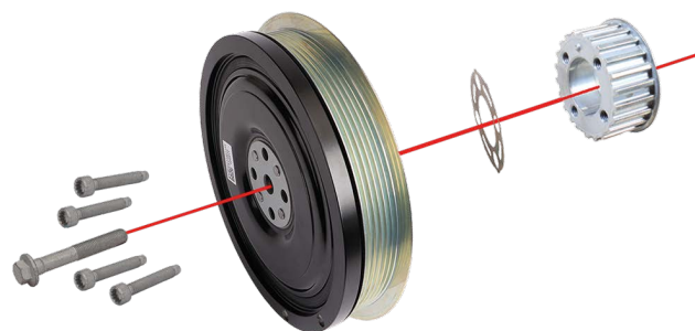
Slika 2: Središnji pričvrtni vijak, četiri pričvrtna vijka pogonske remenice kanalnog remena i dijamantna podložna pločica
