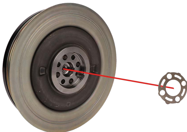
Slika 1: Pogonska remenica kanalnog remena s dijamantnom podložnom pločicom. Nove remenice isporučuju se s podložnom pločicom umetnutom u upuštenje sa stražnje strane pribornice
