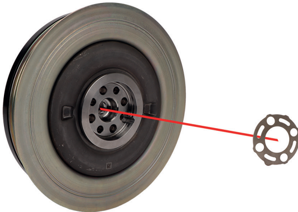
Afbeelding 1: Krukaszijde van de Trillingsdemper krukas met de met diamant bezette drukring. Bij de genoemde KIT's is deze al in de inbouwstand op de Trillingsdemper krukas aangebracht
