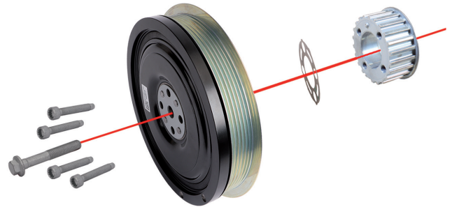
Afbeelding 2: Bouten van de Trillingsdemper krukas, centrale bout van de krukas, Trillingsdemper krukas en met diamant bezette drukring
