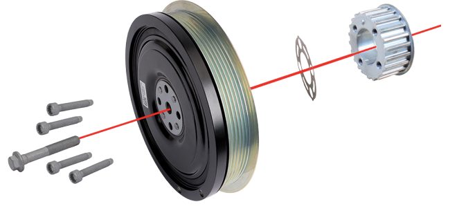
Şekil 2: Titreşim sönümleyicili krank kasnağının civataları, krank milinin merkez civatası, titreşim sönümleyicili krank kasnağı ve özel kaplamalı şim.
