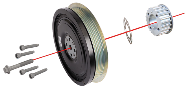
Зображення 2: Гвинти шківів з муфтою вільного ходу, центральний гвинт колінчастого вала, шків з муфтою вільного ходу та підкладна шайба з алмазним покриттям
