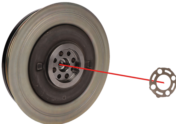
Зображення 1: Бік шківів з муфтою вільного ходу, яким він повернений до колінчастого вала, та підкладна шайба з алмазним покриттям. У наведених вище наборах вона вже вставлена у шків з муфтою вільного ходу і знаходиться у монтажному положенні
