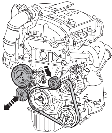
איור 1: מנוע Prince (BMW/PSA)
