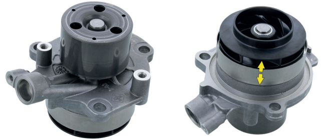
Resim 1: Ayarlanabilir pervane açıklığına sahip 538 0983 10 numaralı su pompası
