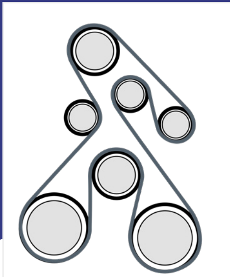
Origineel riemverloop met 2264mm- riem
