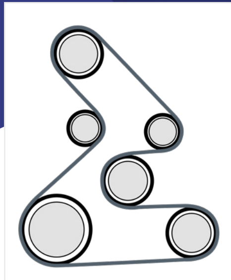
Gewijzigd riemverloop met verwijderde ombuigrol en met 1785mm-riem
